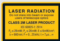
Fig. 3 Laser label and laser warning sign LLT30xx-430, LLT30xx-600
